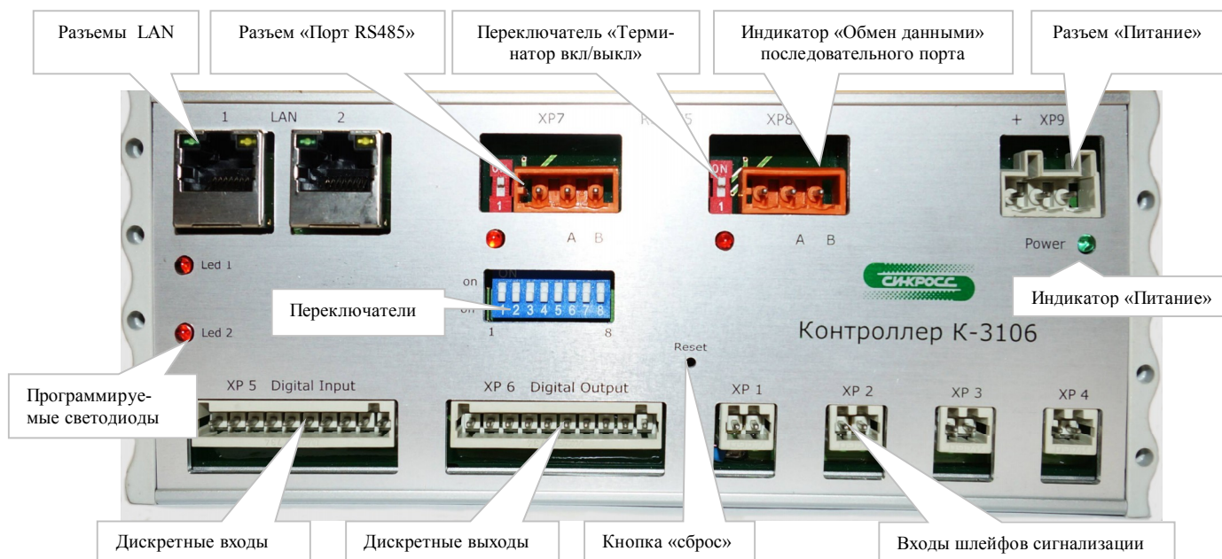
Рисунок В.1. Внешний вид контроллера К-3106
