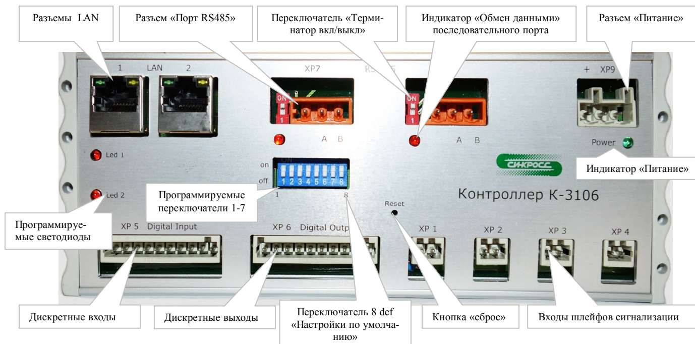
Рисунок 1. Внешний вид контроллера К-3106
