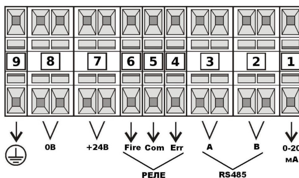
Рисунок 2 – Расположение и назначение клемм модификации ИП 329/330-1-1-Х3ХХ
