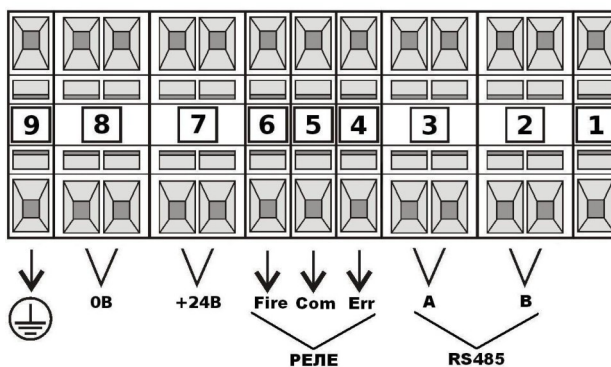
Рисунок 1 – Расположение и назначение клемм модификаций ИП 329/330-1-1-X0XX, ИП 329/330-1-1-X1XX
