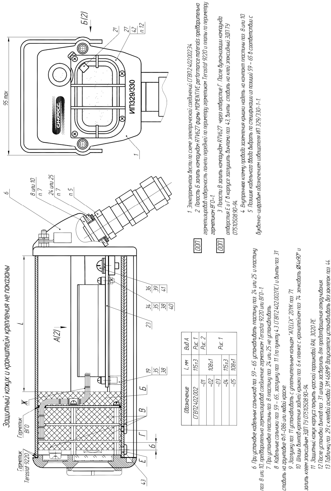
Рисунок Б.1 – Сборочный чертёж
