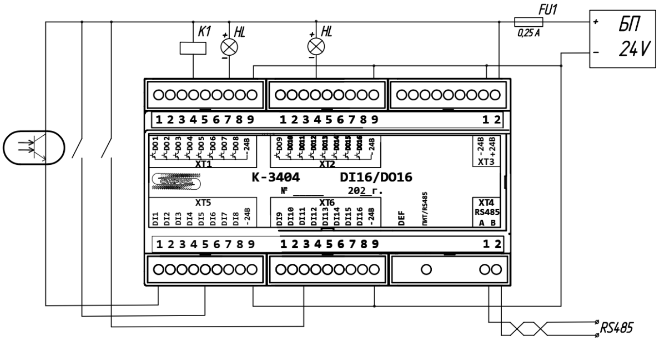
Рисунок А.1 – Схема подключения
