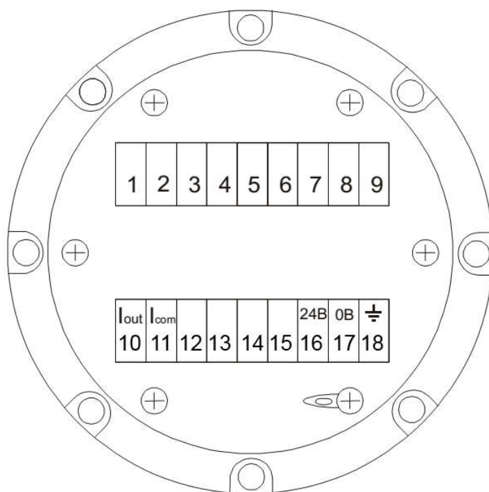
Рисунок 1 - Назначение контактов входных клемм
