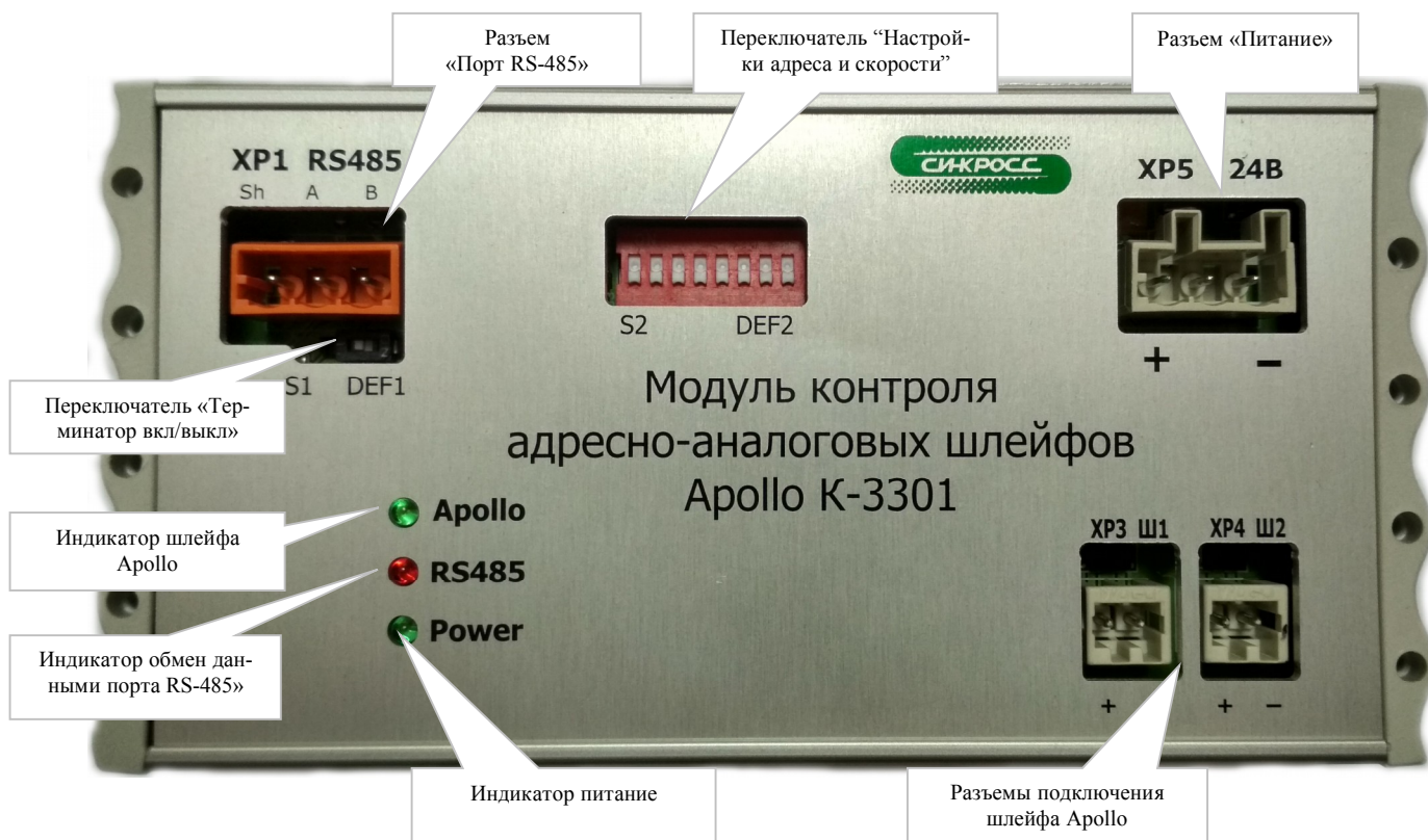
Рисунок 1. Внешний вид модуля K-3301
